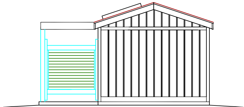
END ELEV.
